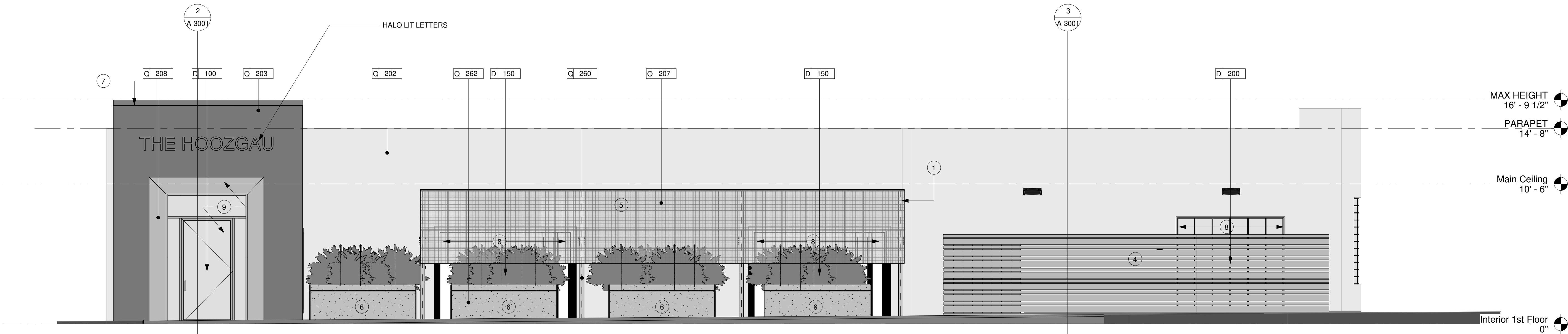
2 NE ELEVATION
